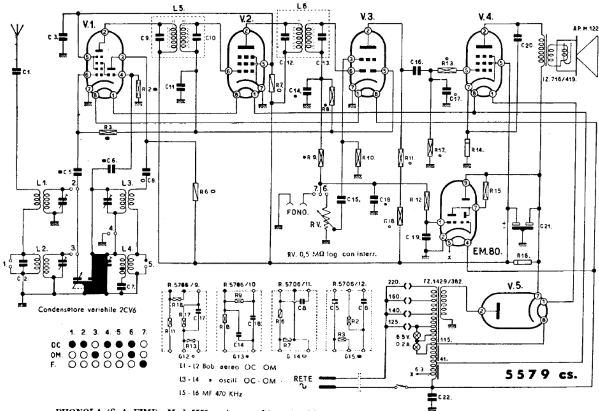
PHONOLA (S. A. FIMI) - Mod. 5579 cs. Apparecchio a circuiti stampati.
